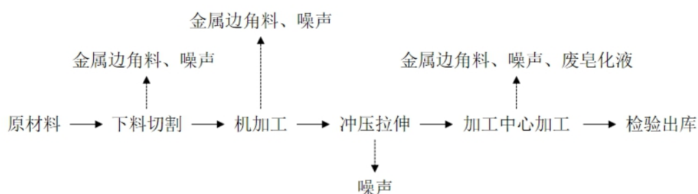
图 3-3 生产工艺流程及产污环节图
